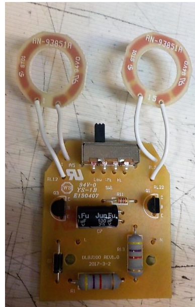
Figura 4. "Aromatizante eléctrico de pared / Componentes internos del producto"
