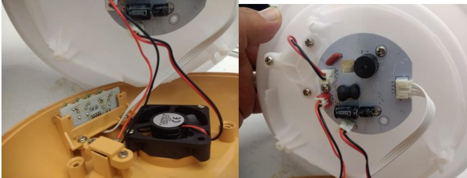
Figura 5. Construcción de un aparato que hace uso de este principio de funcionamiento
